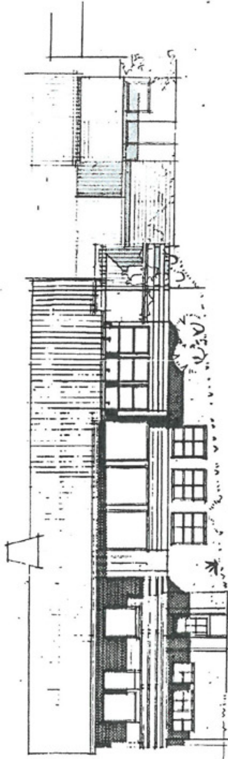
FASADE MOT VEST
